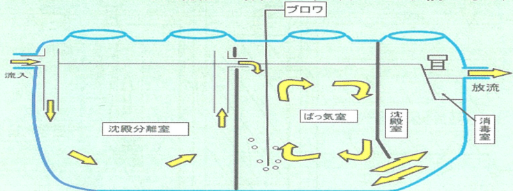
9. みなし浄化槽(分離接触ばっ気方式)
