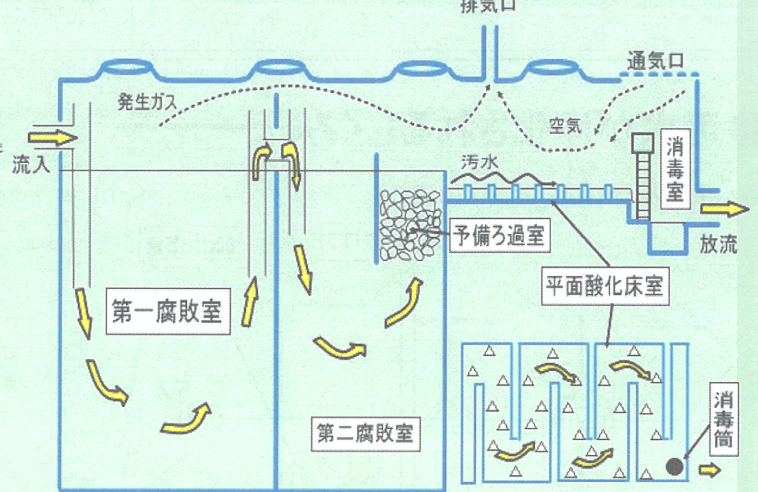
8. みなし浄化槽(散水ろ床方式)
