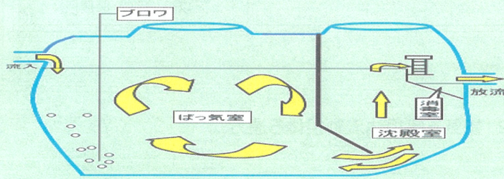
7. みなし浄化槽(分離ばっ気型)
