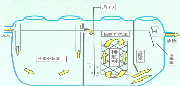
9. みなし浄化槽(分離接触ばっ気方式)
