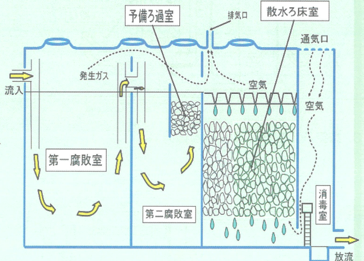
8. みなし浄化槽(散水ろ床方式)
